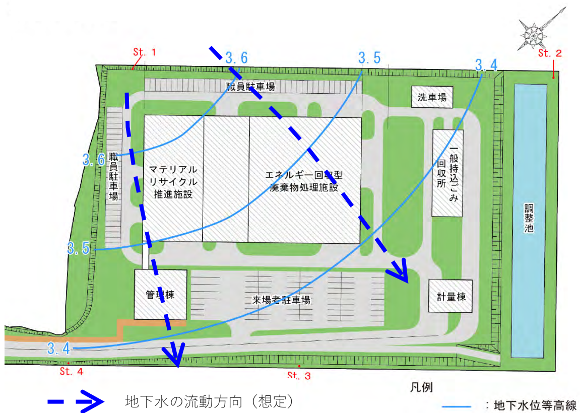
図 7.2.3-6 地下水水位等高線図 (夏季：令和3年8月6日)
