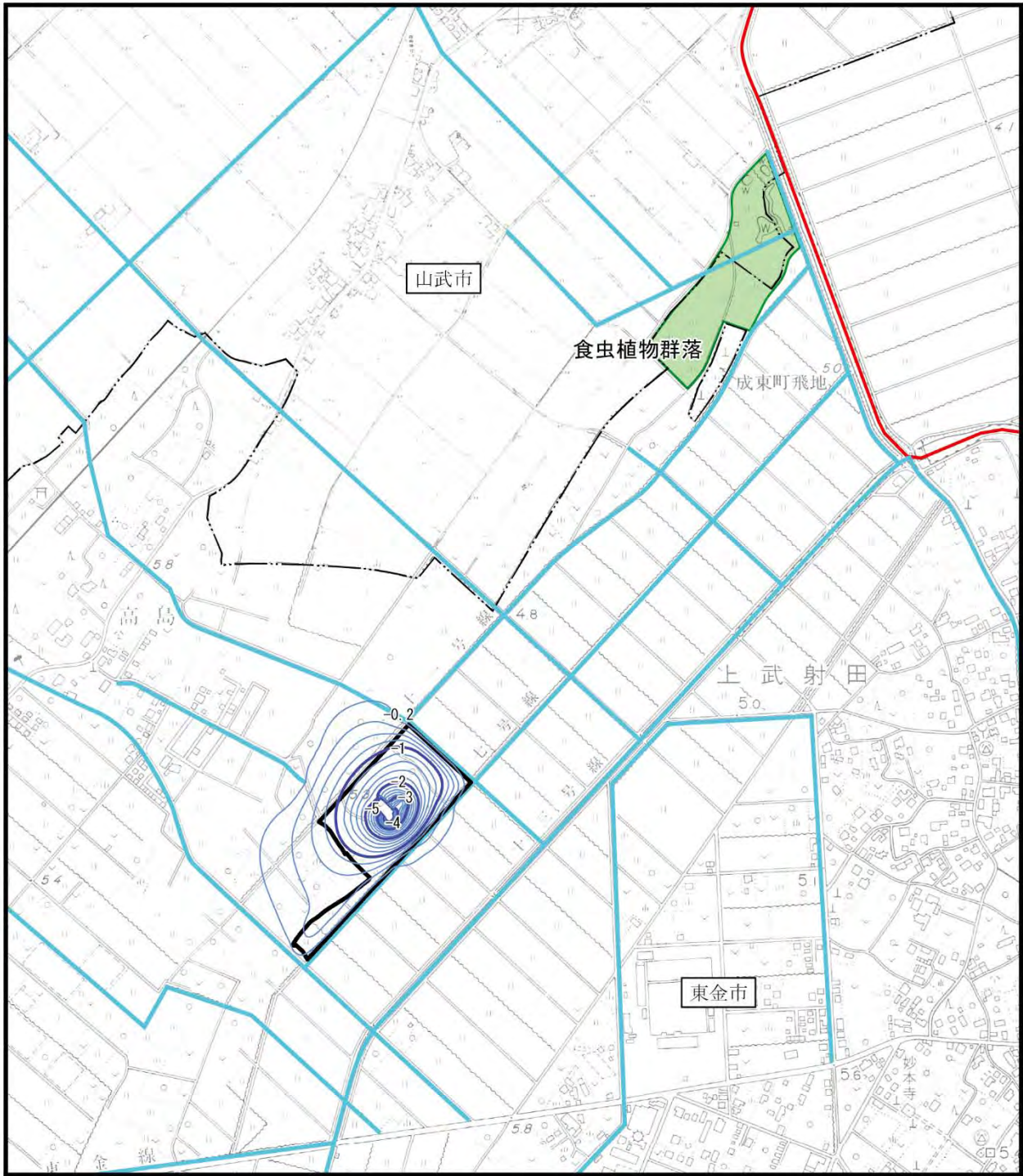
図 7.2.3-11 図 7.2.3-13(1) 地下水位変化量予測結果【工事中】 (調整池の工事後+工場棟の工事中/灌漑期)
