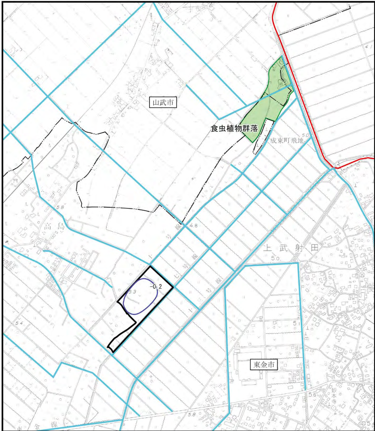
図 7.2.3-14 図 7.2.3-16(2) 地下水位変化量予測結果【完了後】 (非灌漑期)
