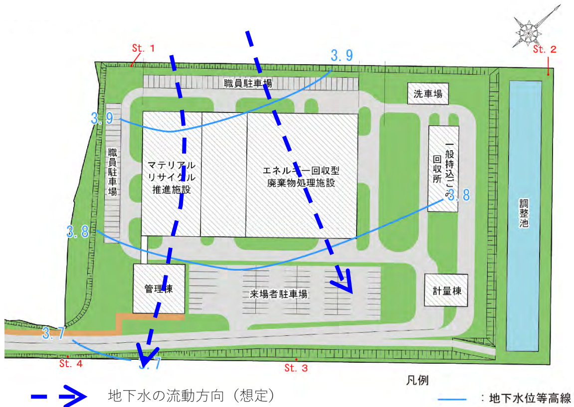
図 7.2.3-5 地下水水位等高線図 (春季：令和3年5月12日)
