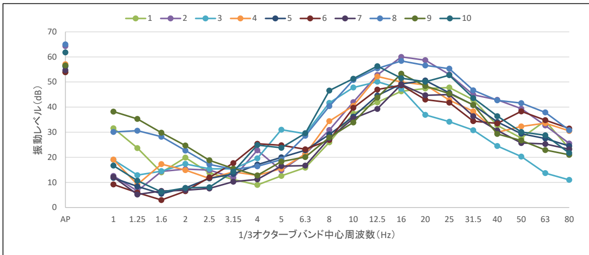
図 6.3-1(1) 地盤卓越振動数調査結果 (St.1)
