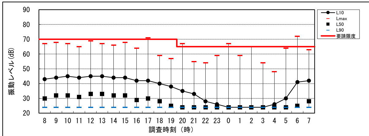
図 6.1-2(5) 道路交通振動調査結果 (St.2、休日)
