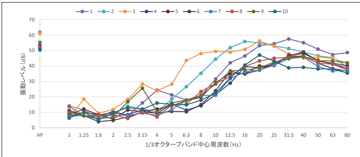
図 6.3-1(2) 地盤卓越振動数調査結果 (St.2)
