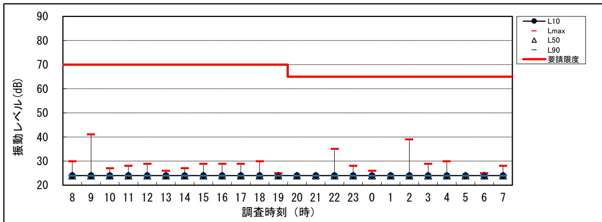
図 6.1-1(3) 環境振動調査結果 (St.3)
