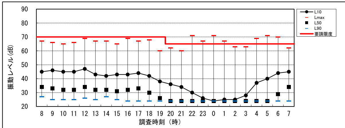
図 6.1-2(4) 道路交通振動調査結果 (St.2、平日)
