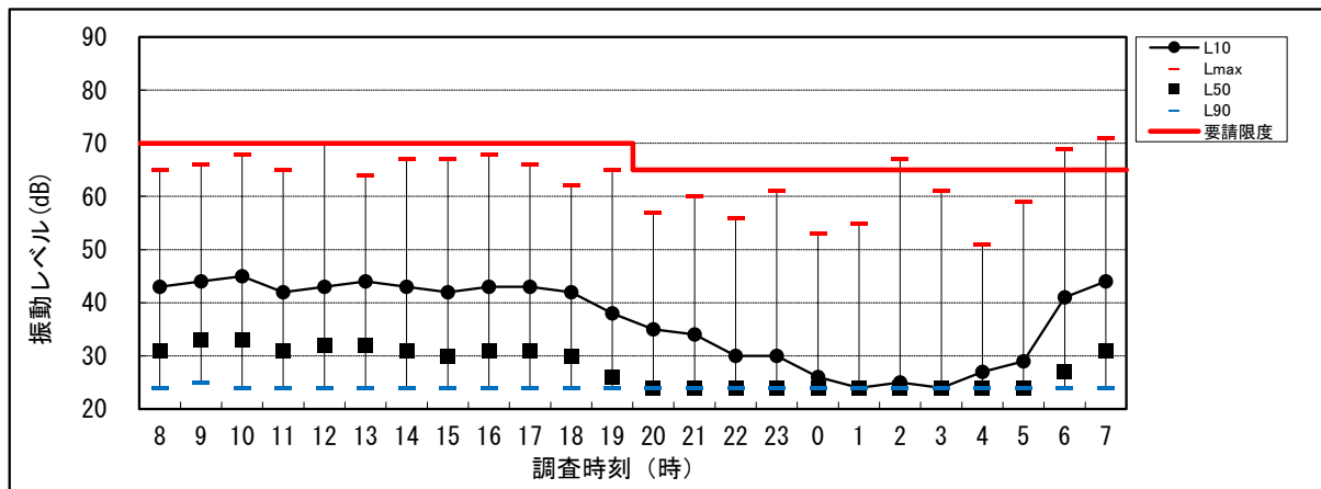
図 6.1-2(6) 道路交通振動調査結果 (St.2、夏季)
