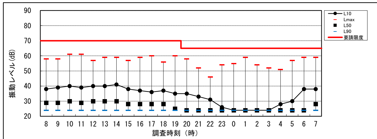
図 6.1-2(2) 道路交通振動調査結果 (St.1、休日)
