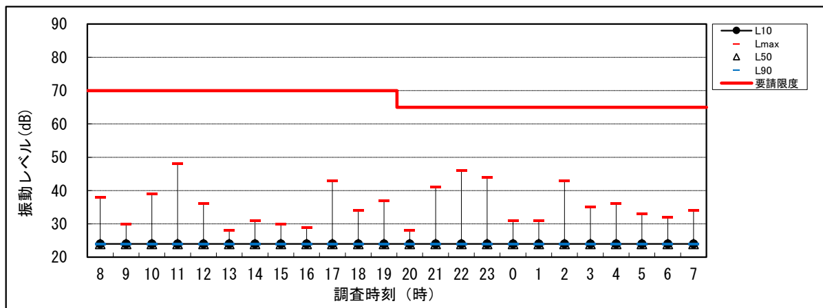
図 6.1-1(4) 環境振動調査結果 (St.4)
