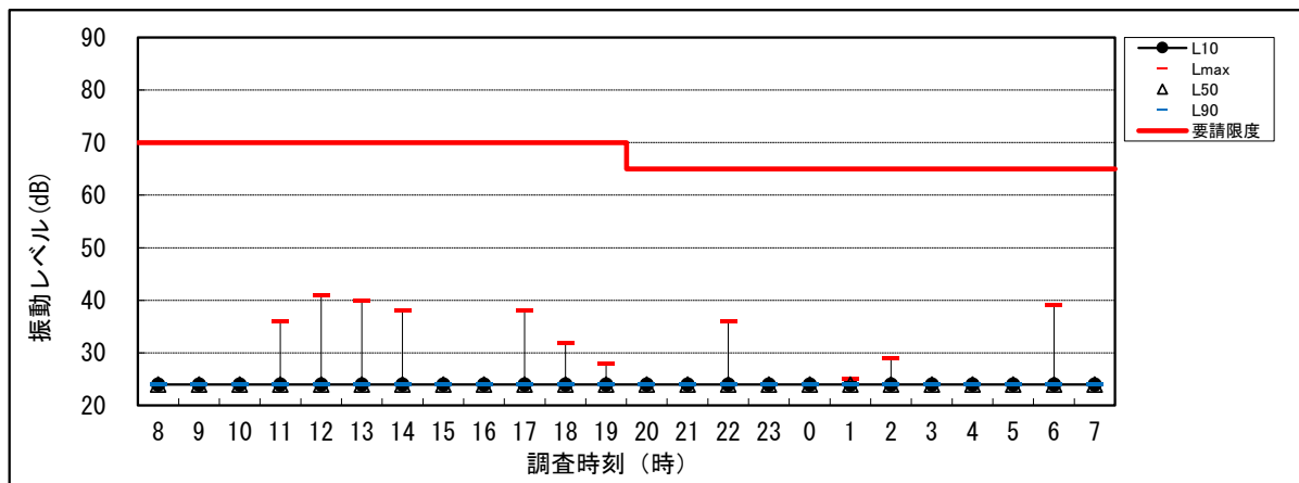
図 6.1-1(1) 環境振動調査結果 (St.1)
