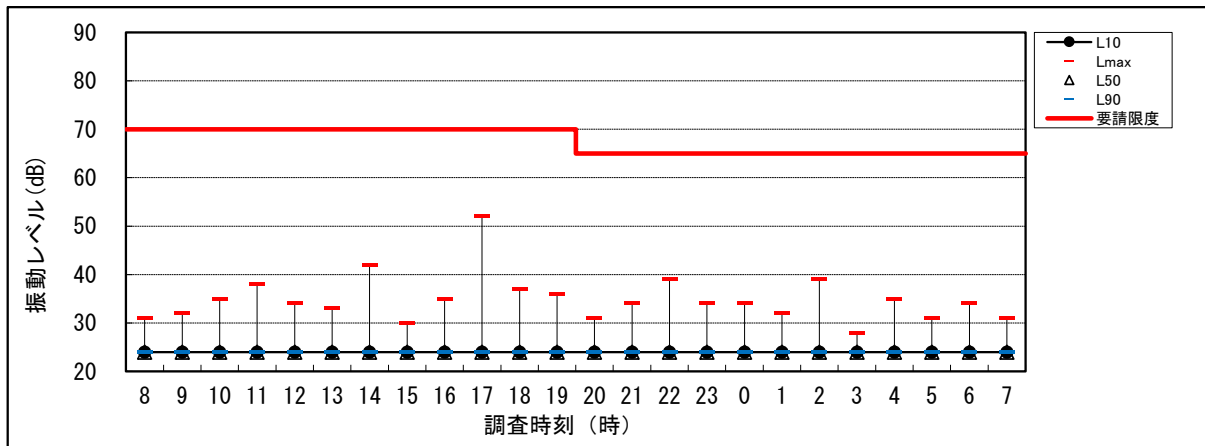
図 6.1-1(2) 環境振動調査結果 (St.2)
