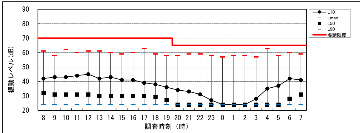
図 6.1-2(1) 道路交通振動調査結果 (St.1、平日)
