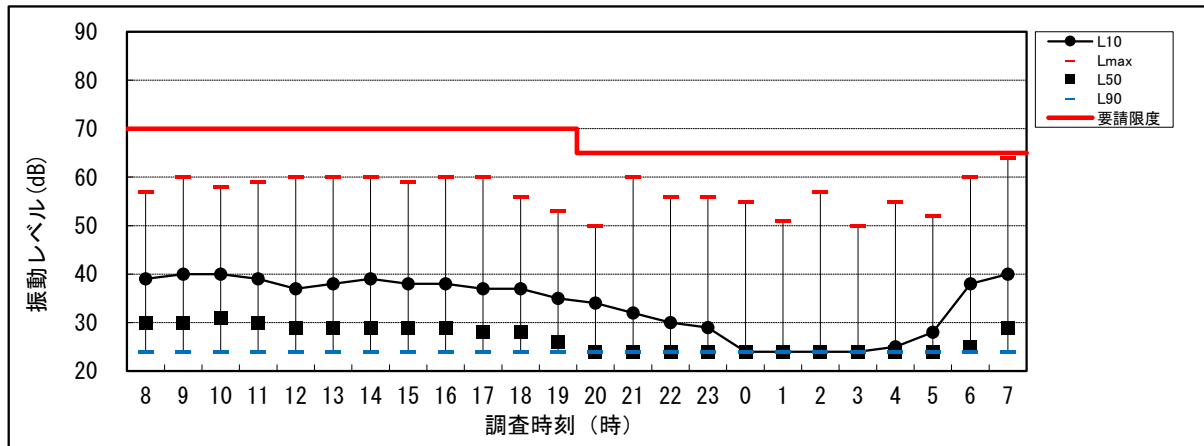
図 6.1-2(3) 道路交通振動調査結果 (St.1、夏季)
