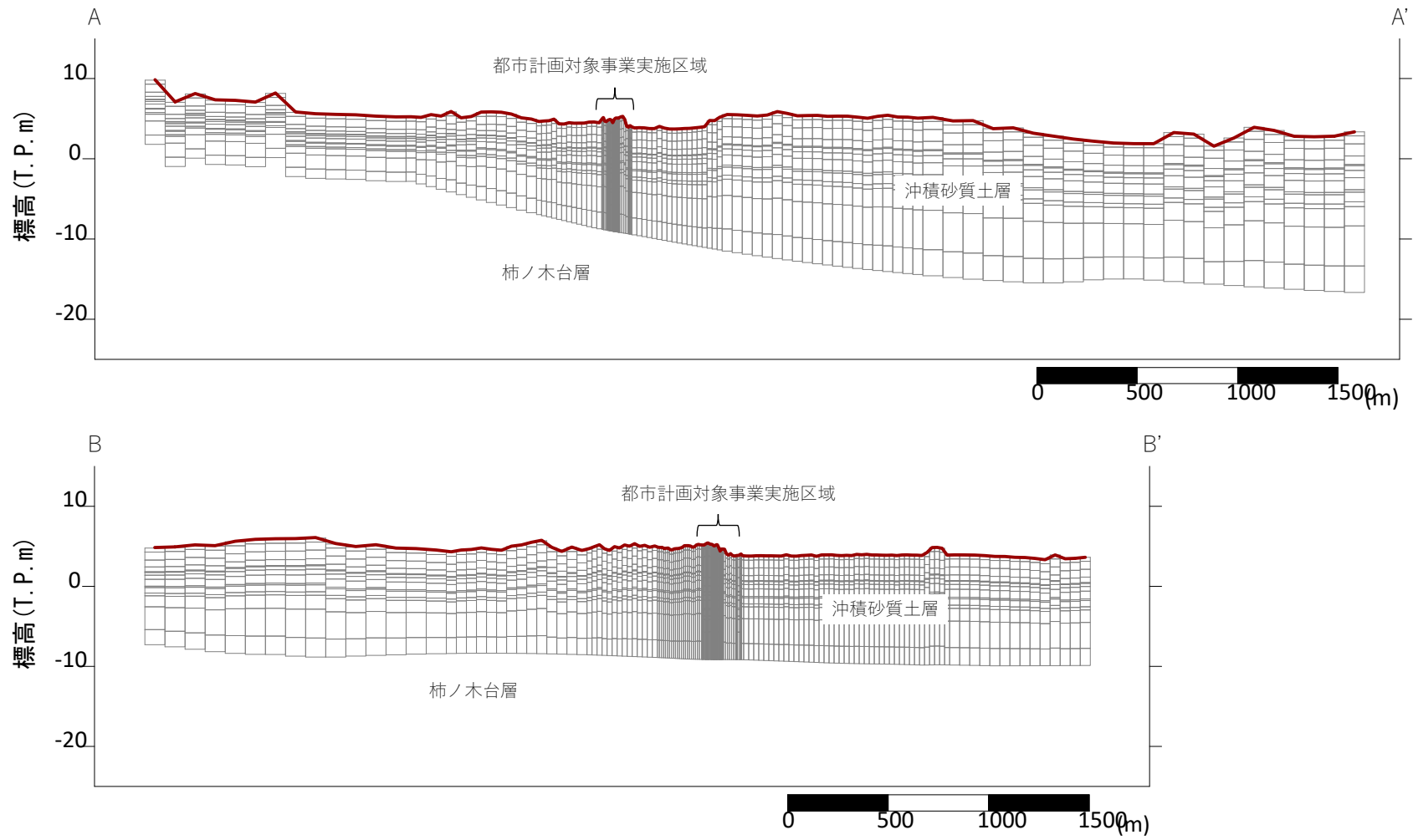
図 4.1-2 地下水解析モデルにおける解析メッシュ (代表断面)
