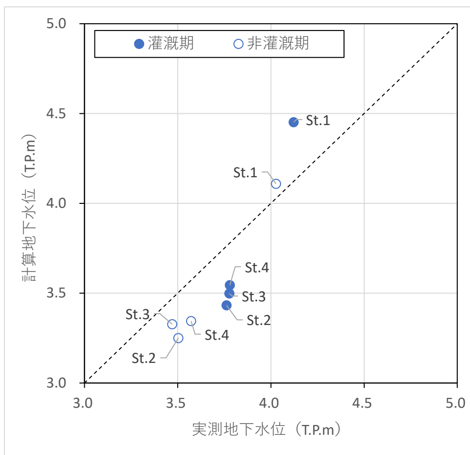
図 4.1-6 地下水位の再現性検証結果 (地下水位観測井戸 St.1～4)
