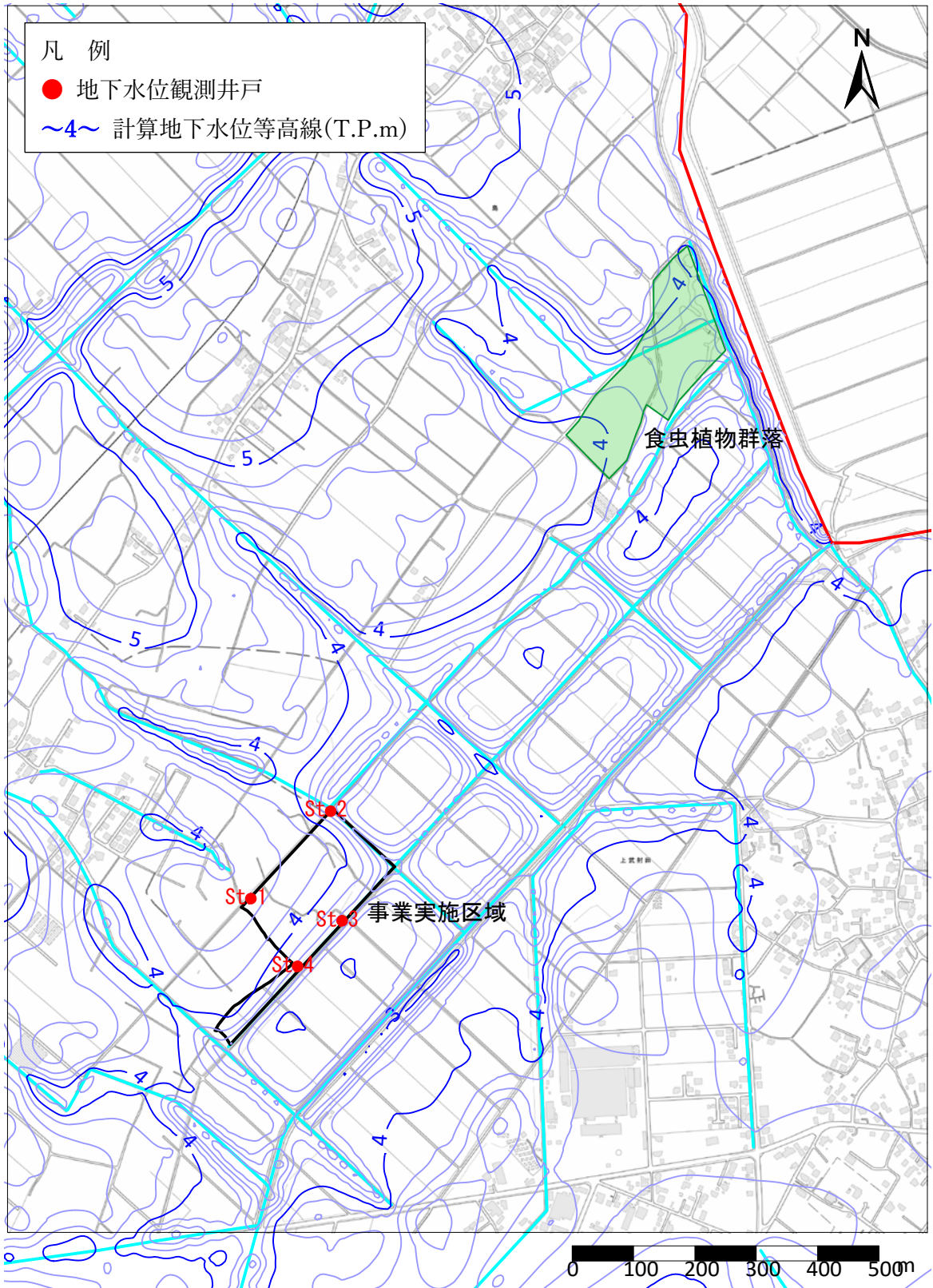
図 4.1-7(1) 計算地下水位分布（灌漑期）
