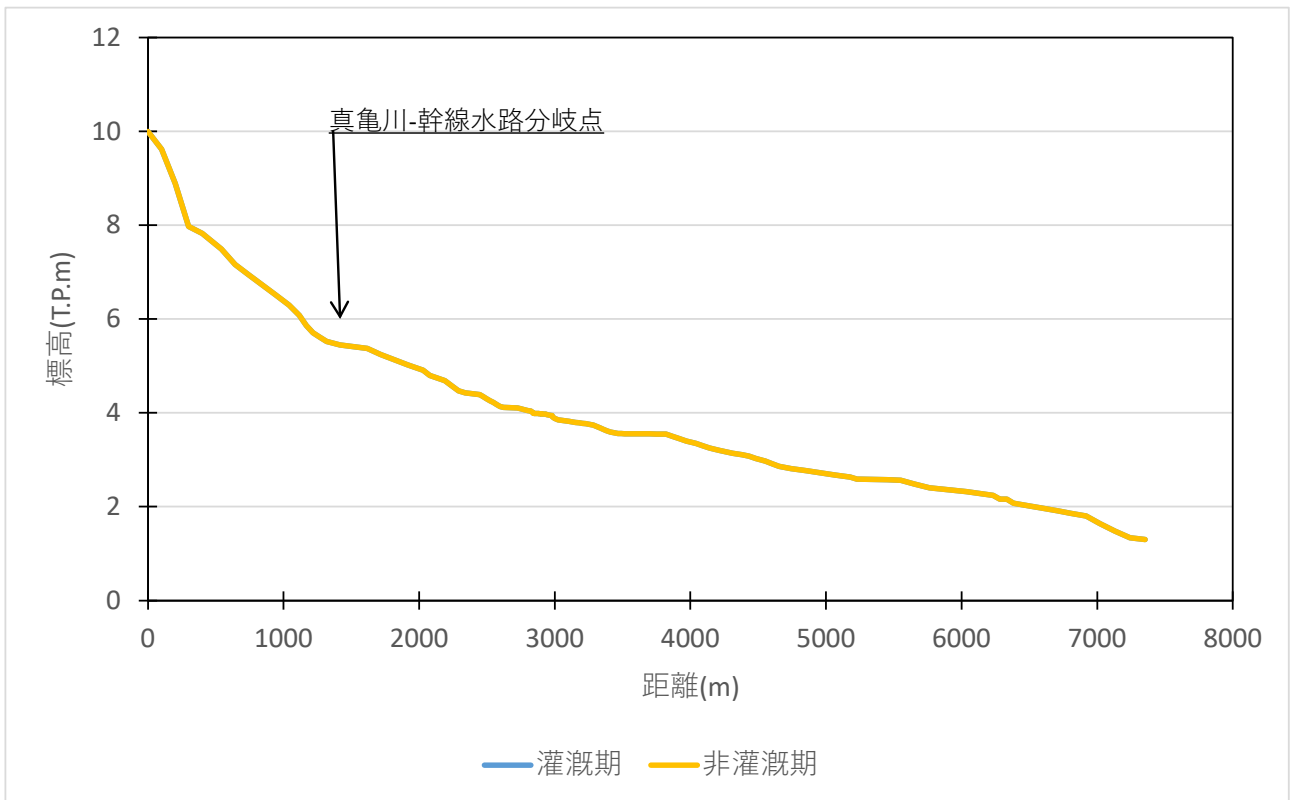
図 4.1-3 固定水頭境界 (河川・水路) に設定した河川水位
