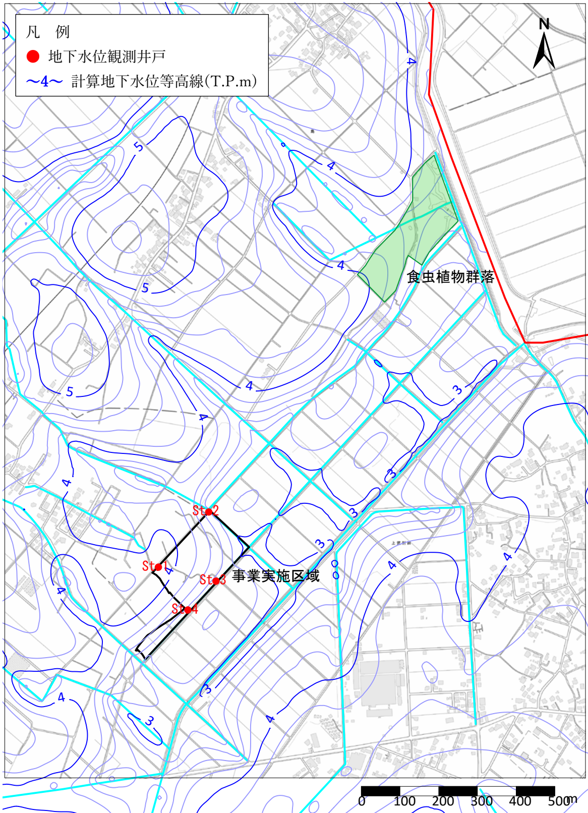
図 4.1-7(2) 計算地下水位分布 (非灌漑期)
