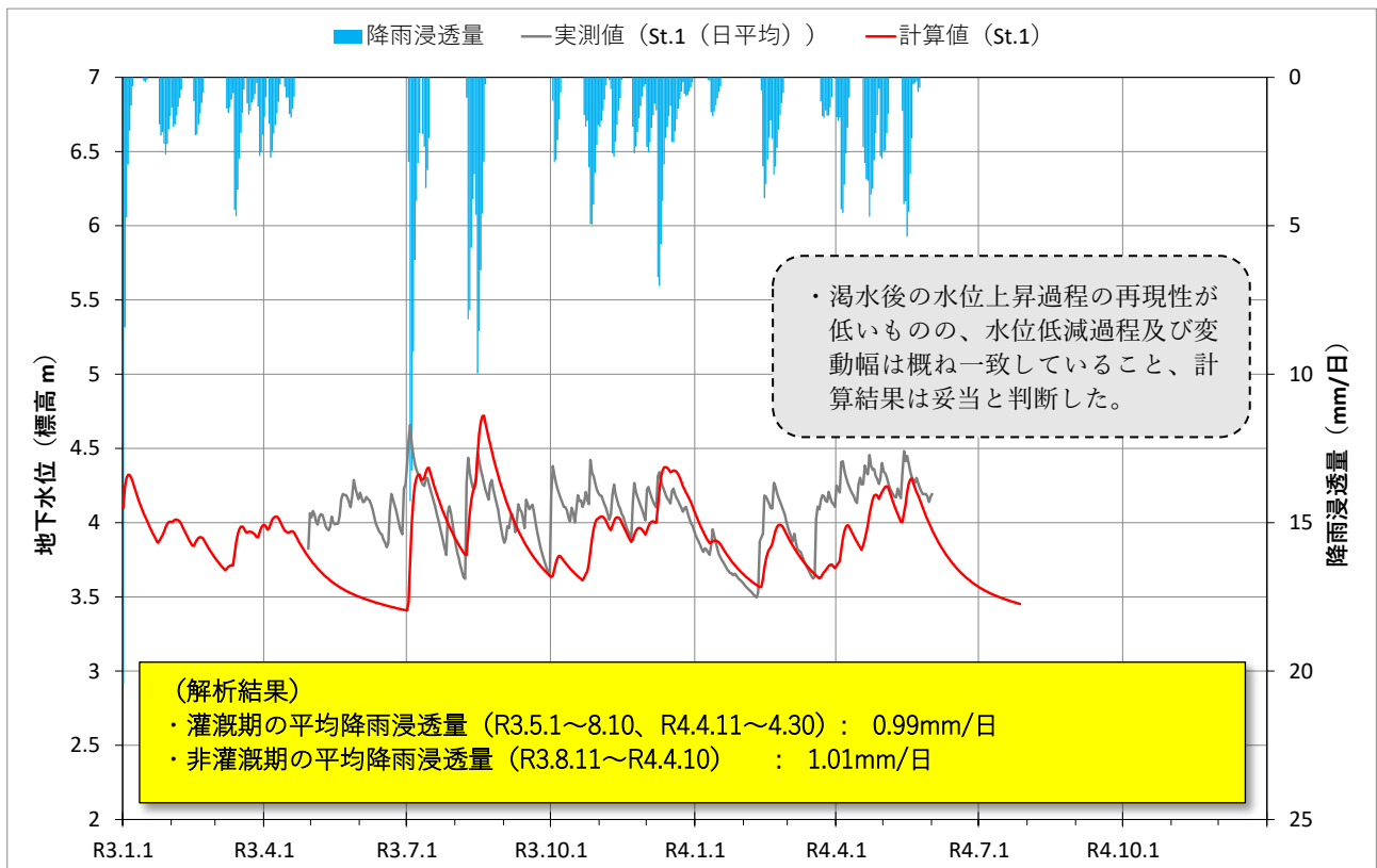
図 4.1-5 タンクモデル法による降雨浸透量の推定
