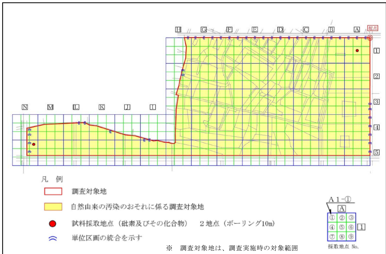
図 7.2.9-2(2) 土壌汚染調査地点（自然由来汚染調査）
