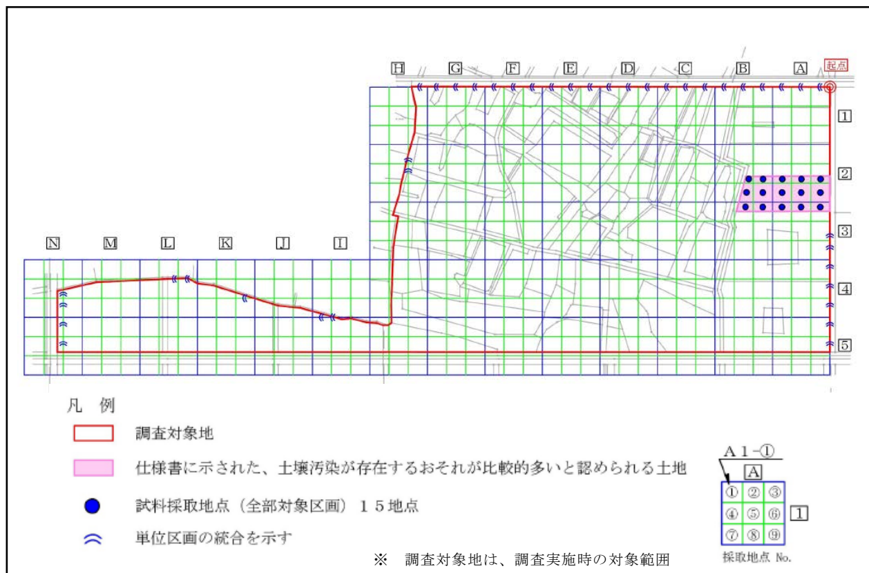
図 7.2.9-2(1) 土壌汚染調査地点（人為等由来汚染調査）
