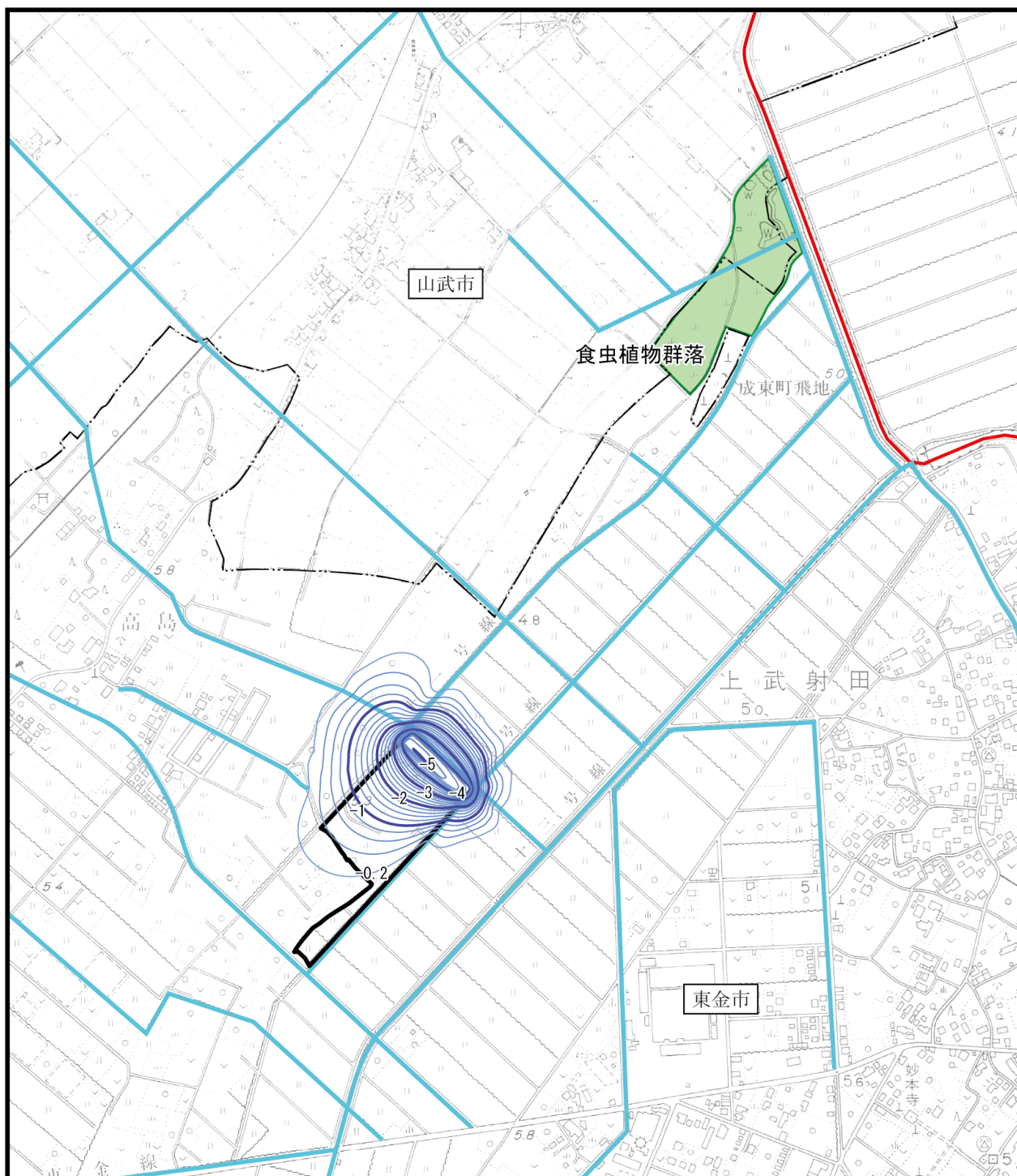
図 7.2.3-12(1) 地下水位変化量予測結果【工事中】 (調整池の工事中／灌漑期)
