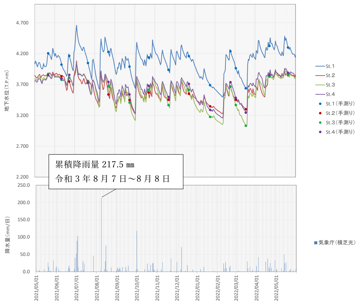
図 7.2.3-5 地下水位の状況（不圧地下水）
