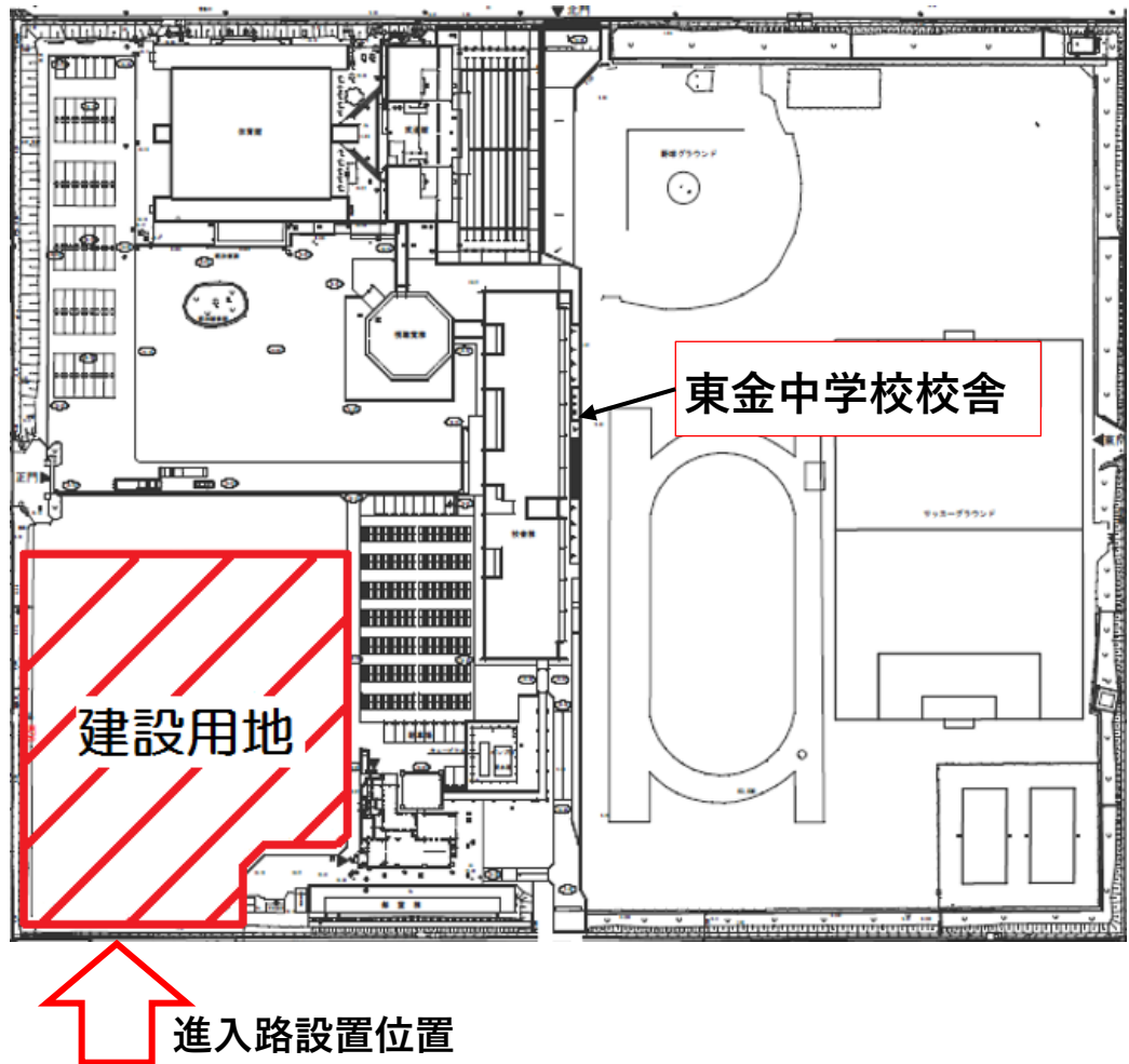
【図2 形状図】
